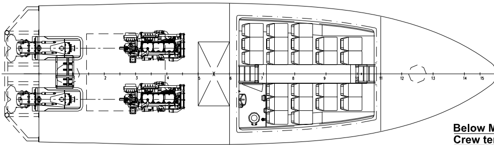
Maindeck
